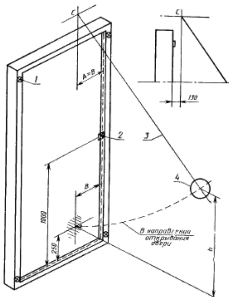
1 — прижим; 2 — зажимающий прибор или ограничитель; 3 — гибкая нить; 4 — неупругое тело (груз). B = \frac{1}{2} ширины полотна, но не более 300 мм.
